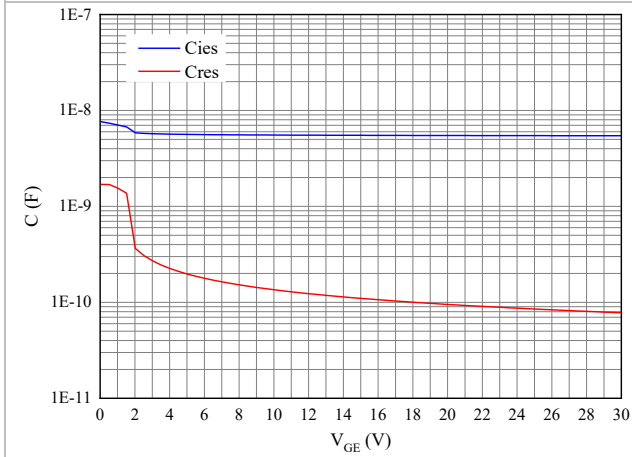
图 9. 电容特性
