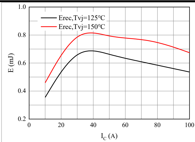
图 7. 开关损耗 二极管
